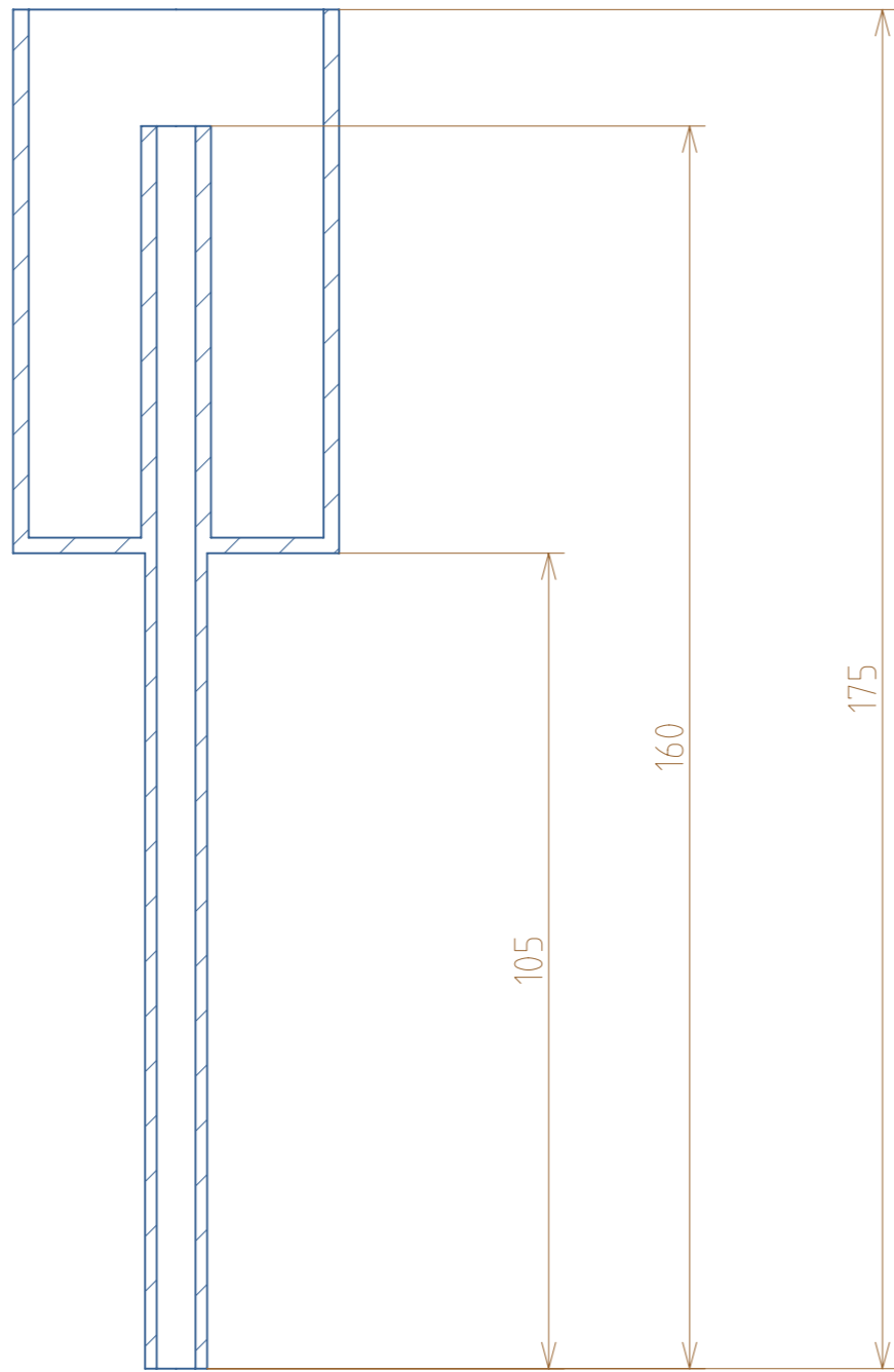
SECTION A-A
