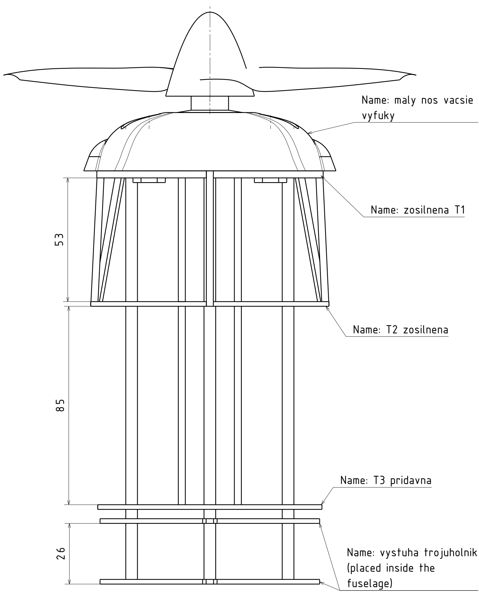
Front view Scale: 1:1
