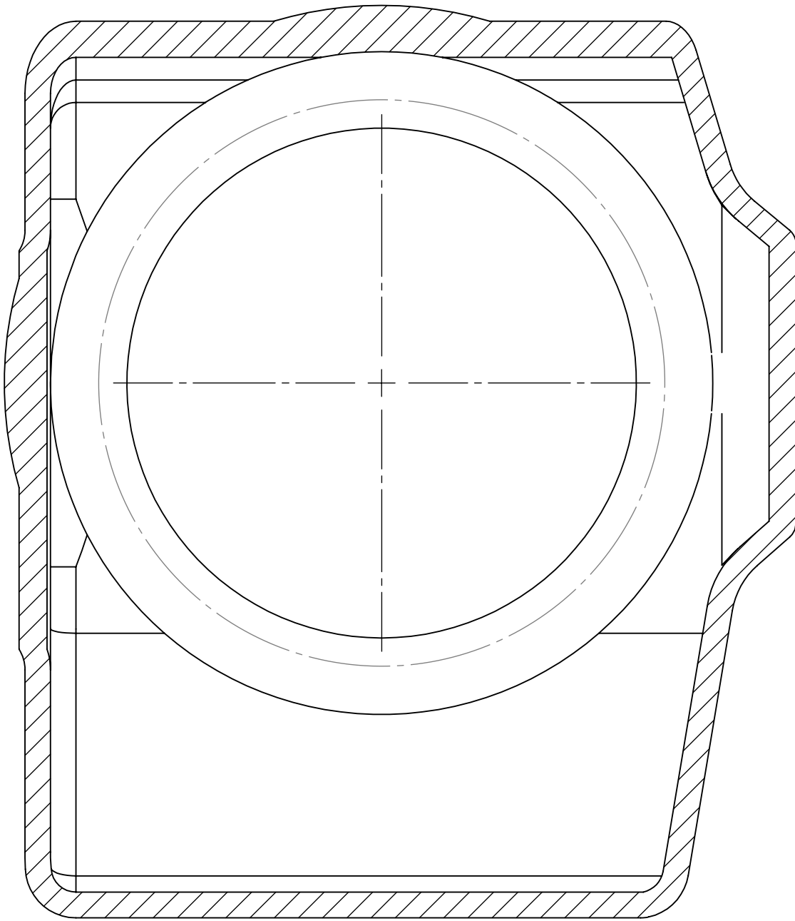
SECCIÓN 9-9 ESCALA 1 : 1
