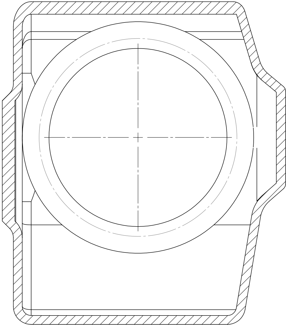
SECCIÓN 8-8 ESCALA 1 : 1
