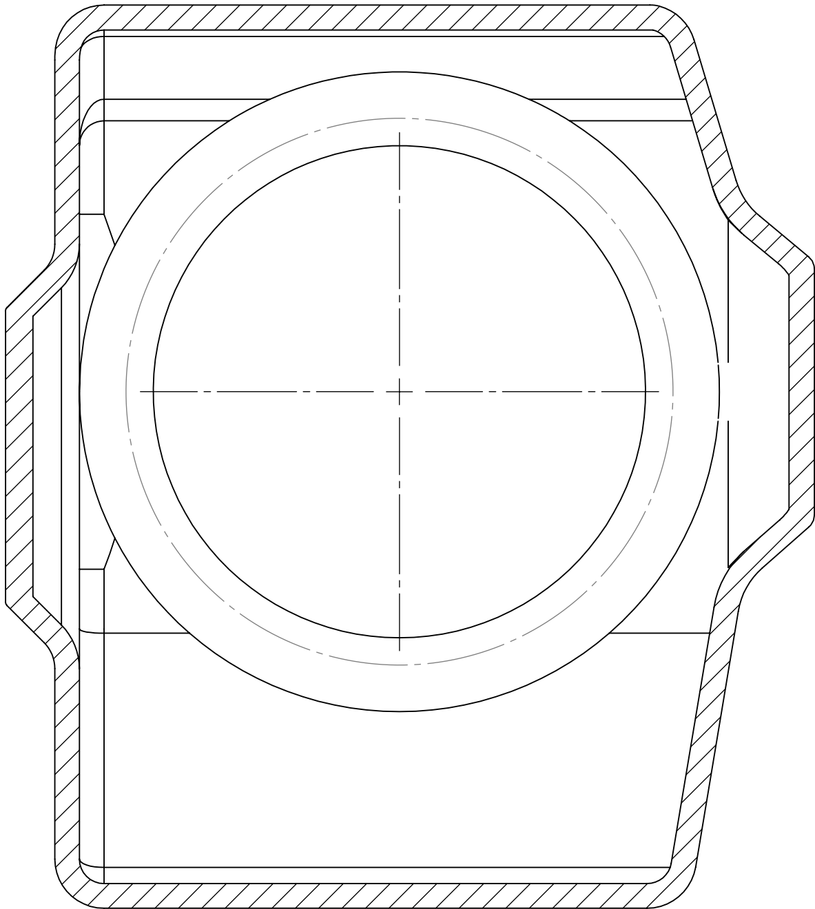
SECCIÓN 7-7 ESCALA 1 : 1
