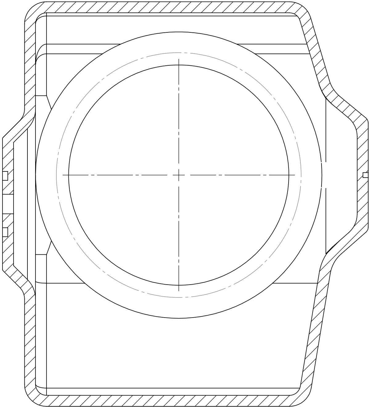
SECCIÓN 5-5 ESCALA 1 : 1
