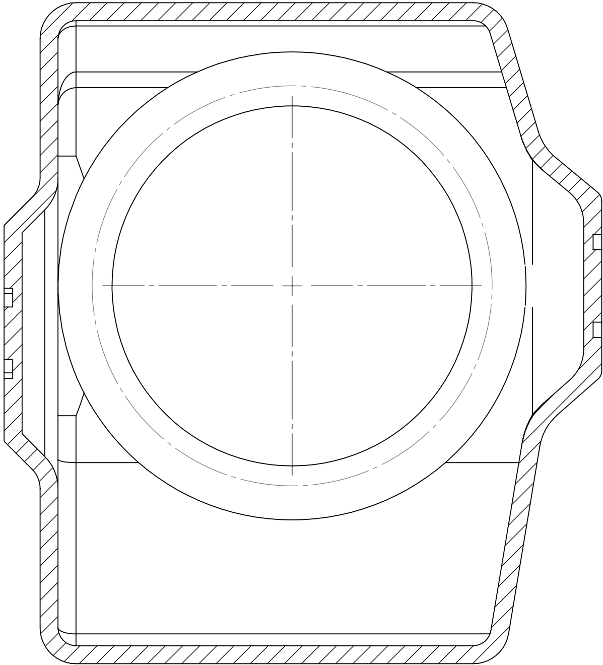
SECCIÓN 4-4 ESCALA 1 : 1
