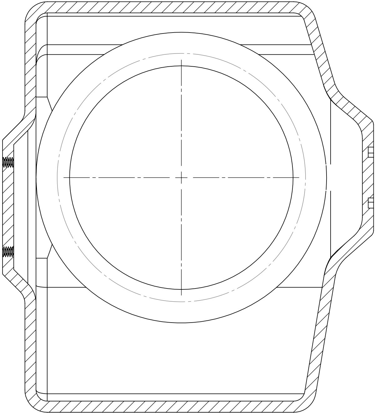
SECCIÓN 3-3 ESCALA 1 : 1
