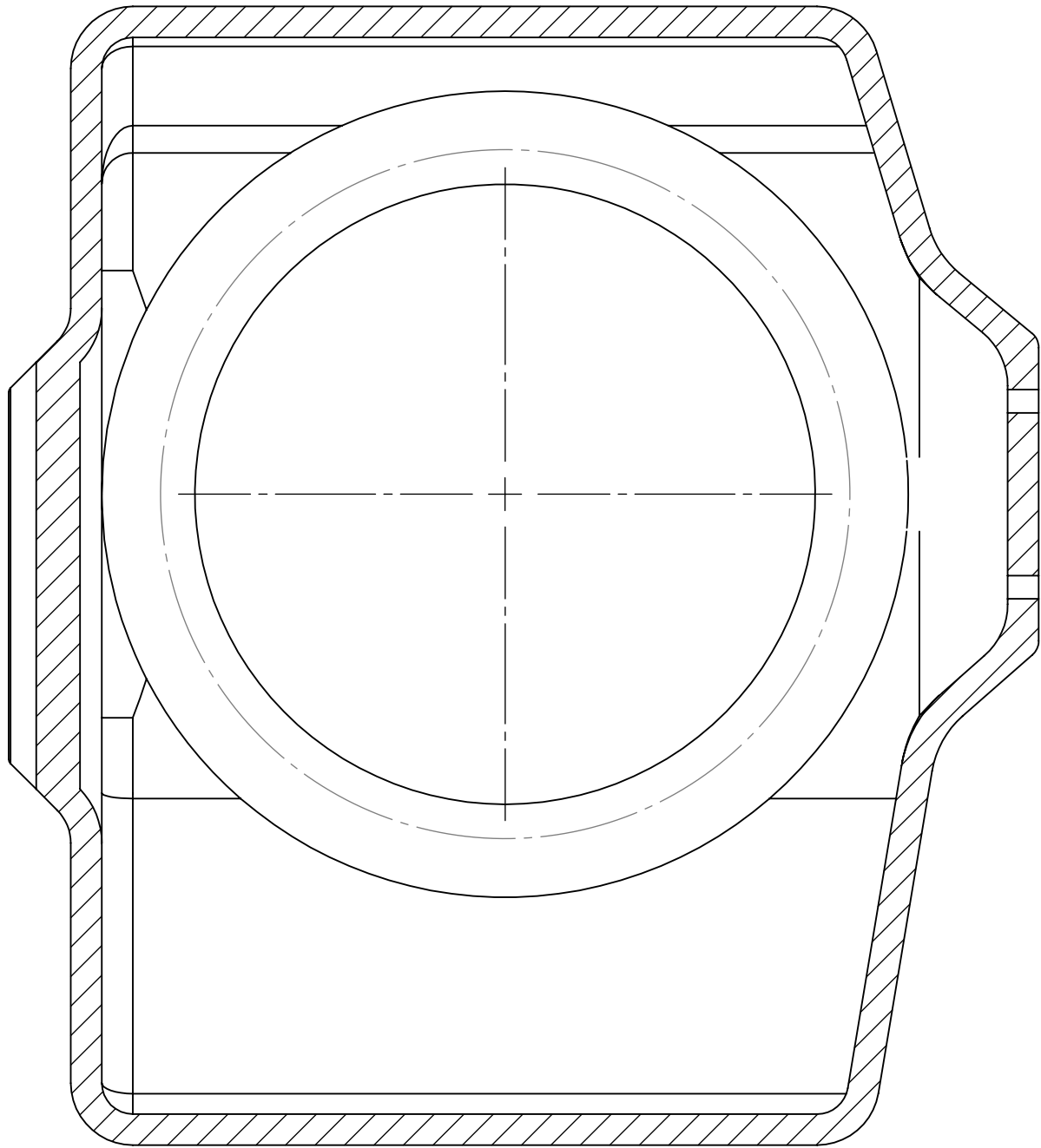
SECCIÓN 2-2 ESCALA 1 : 1
