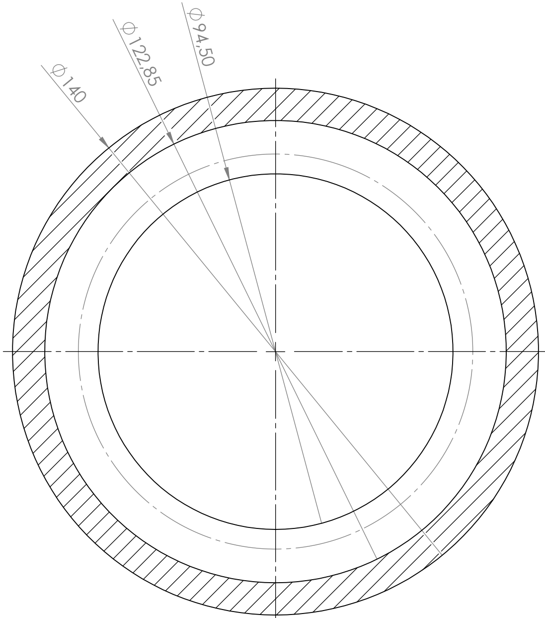
SECCIÓN 14-14 ESCALA 1 : 1
