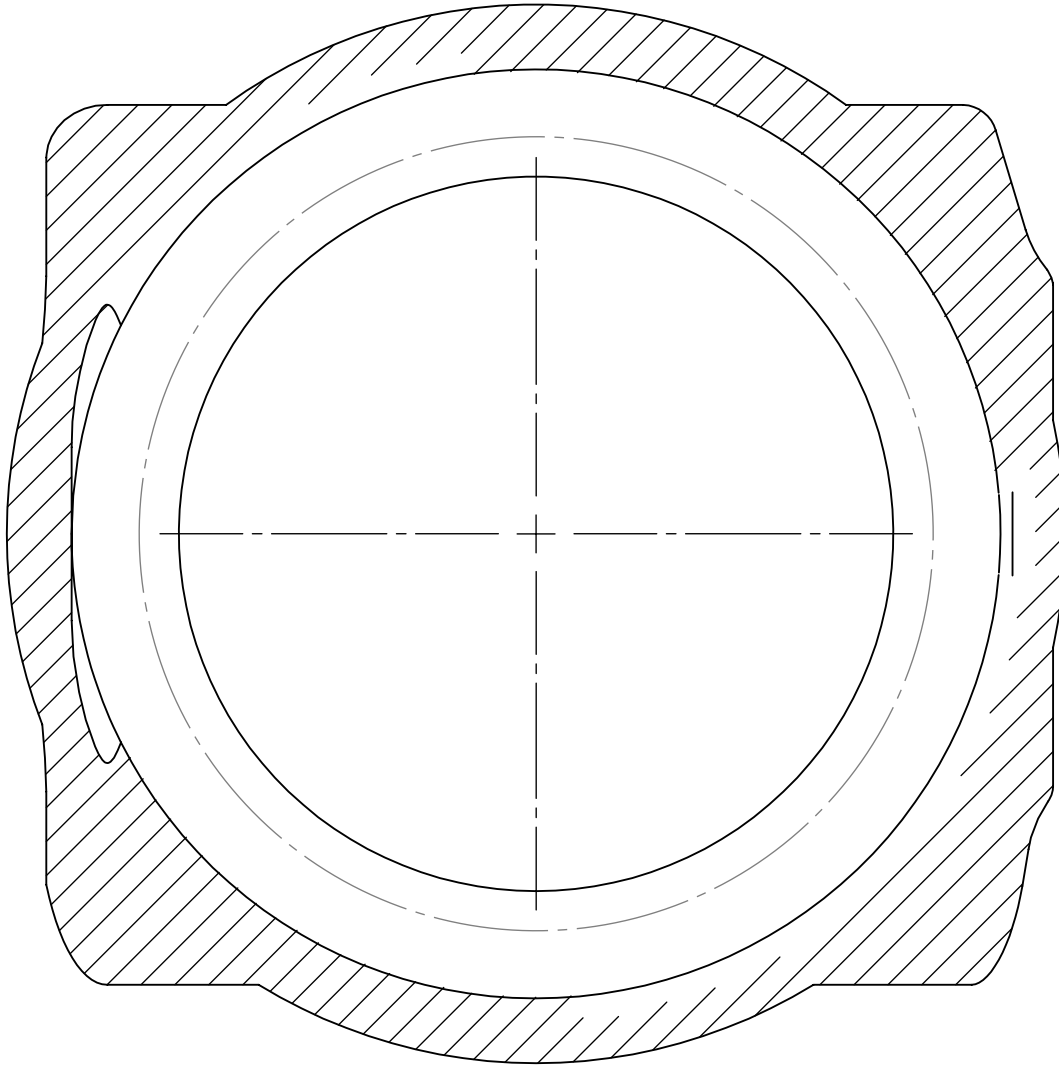
SECCIÓN 13-13 ESCALA 1 : 1
