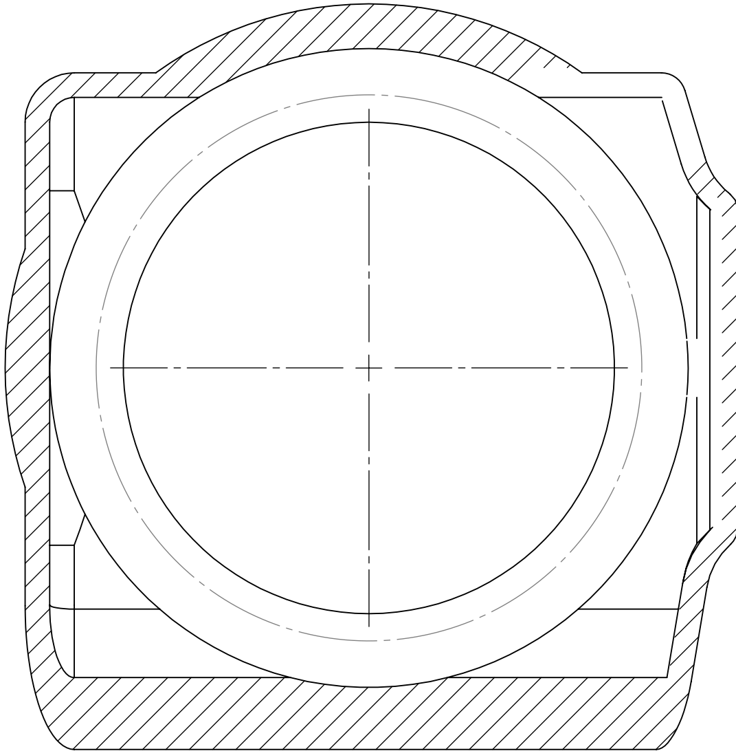
SECCIÓN 12-12 ESCALA 1 : 1
