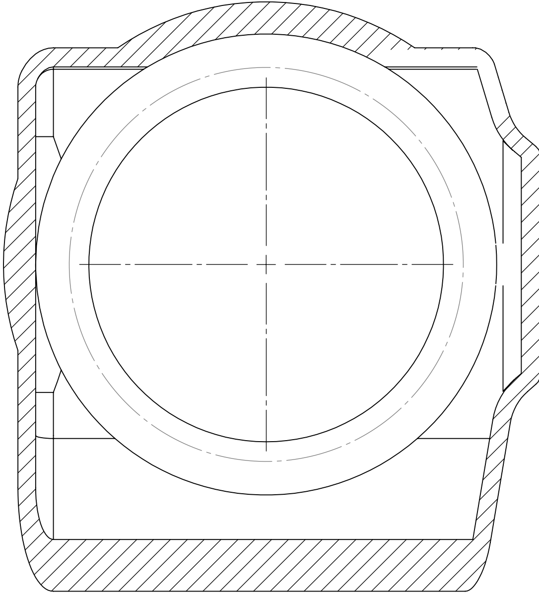
SECCIÓN 11-11 ESCALA 1 : 1
