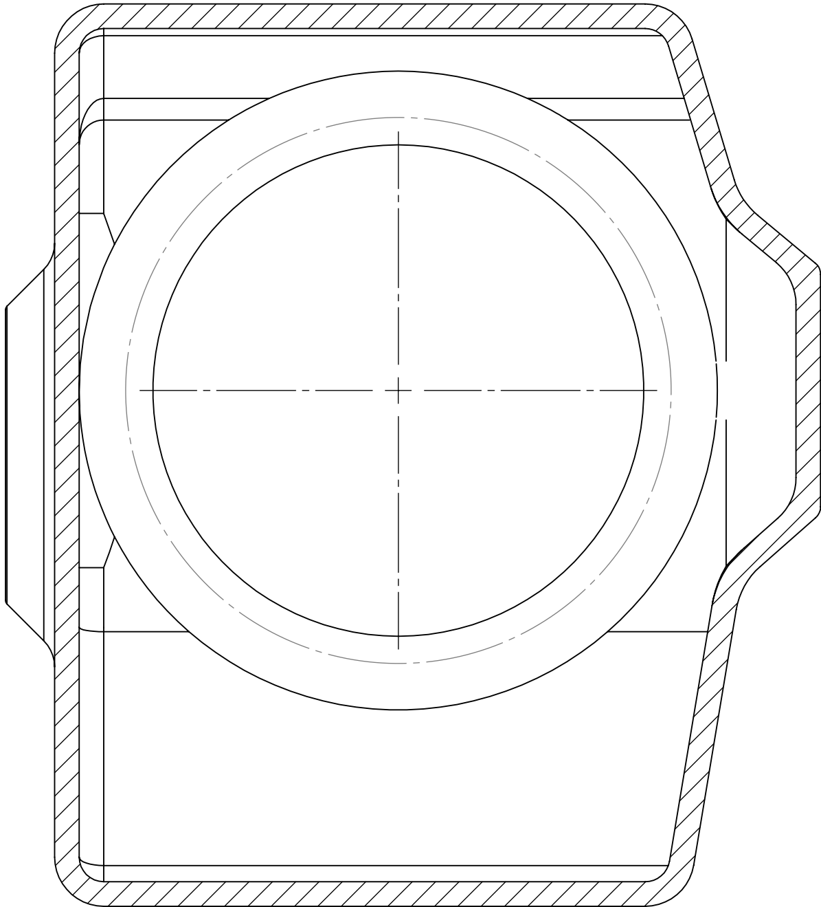
SECCIÓN 1-1 ESCALA 1 : 1
