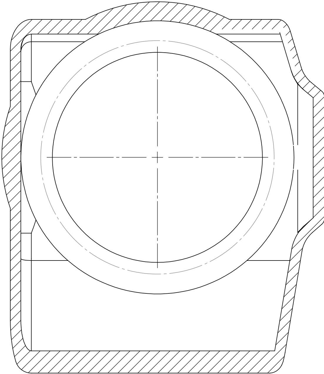
SECCIÓN 10-10 ESCALA 1 : 1
