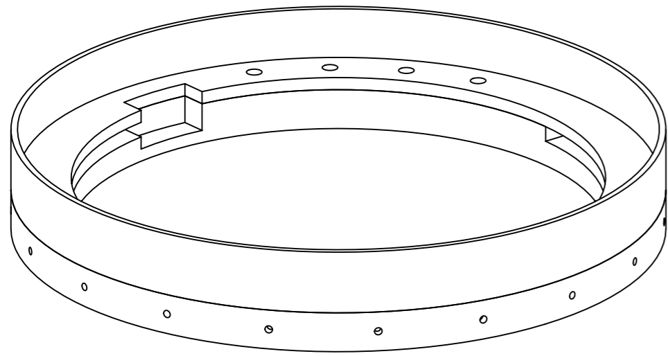
Bovenplaat 1 & 2 Schaal: 1:5
