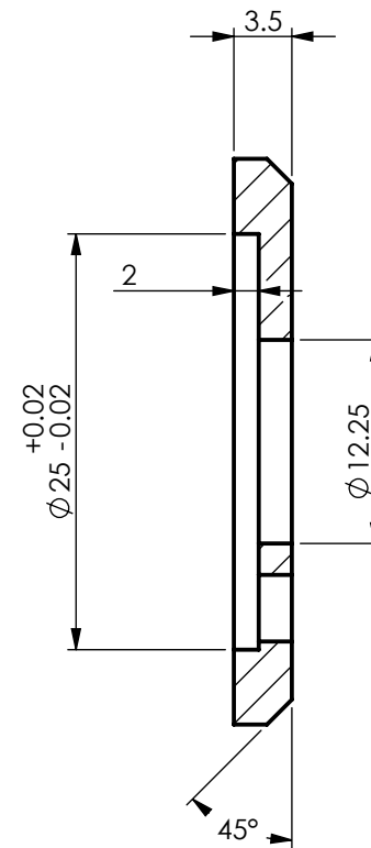
SECTION V-V
