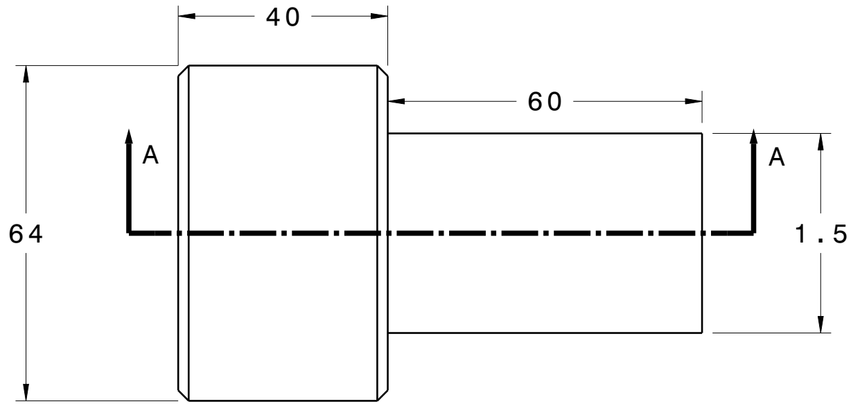
Right view Scale: 1:1
