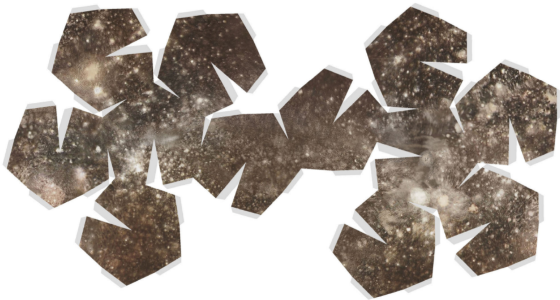
SATELITE DE JUPITER CALISTO
