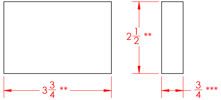
SLIDER 1X
