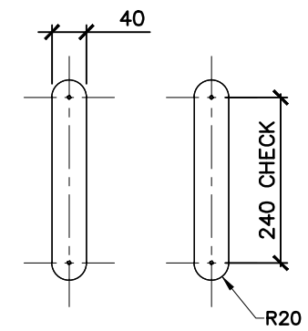
HINGE ARMS
